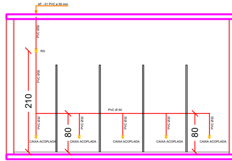
ISOMÉTRICA AF - 01 SANITÁRIO Escala 1/25
