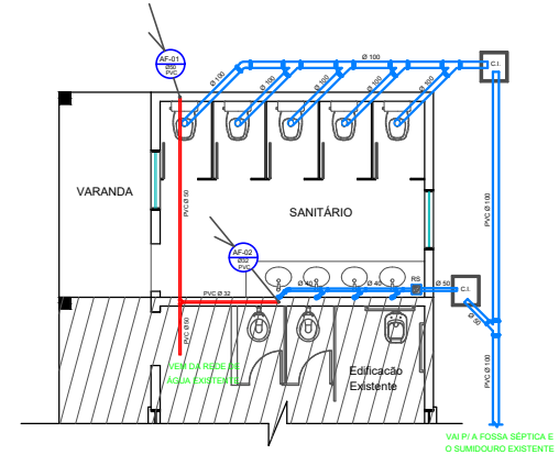
Esquema Hidrosanitário Bloco Serviços Escala 1/50
