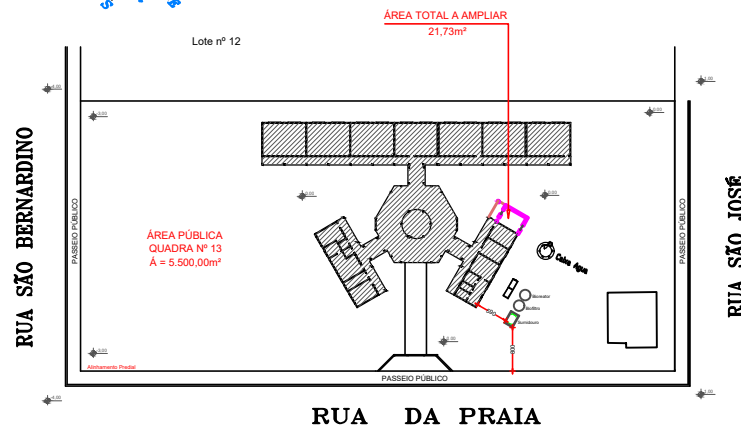
Planta De Locação Biofiltro / Bioreator / Sumidouro Escala 1/500
