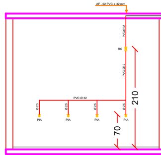
ISOMÉTRICA AF - 02 SANITÁRIO Escala 1/25
