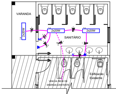
Esquema Elétrico Bloco Serviços Escala 1/50
