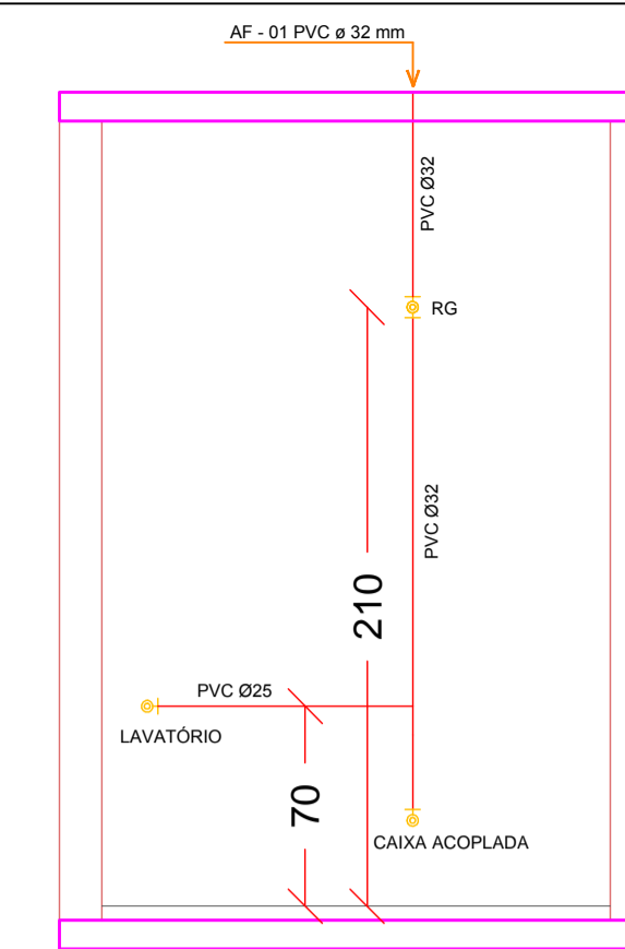
ISOMÉTRICA AF - 01 WC Escala 1/25
