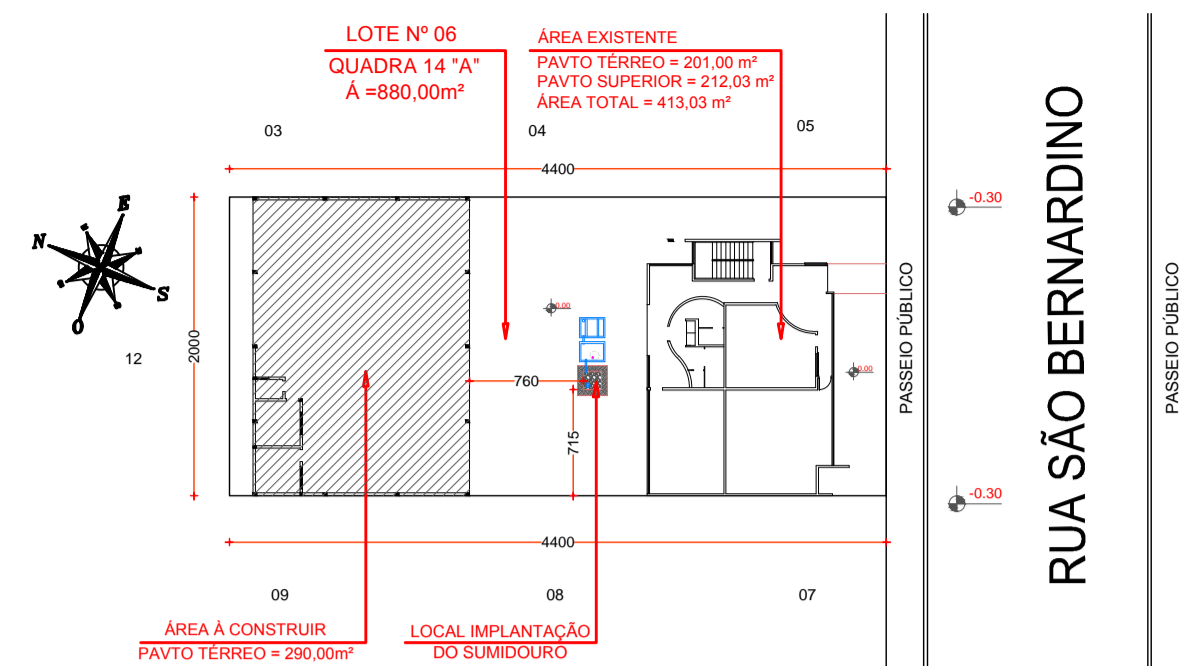
Planta De Localização Do Sumidouro Existente Escala 1/500
