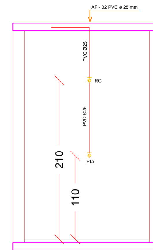
ISOMÉTRICA AF - 02 PIA SALA 02 Escala 1/25
